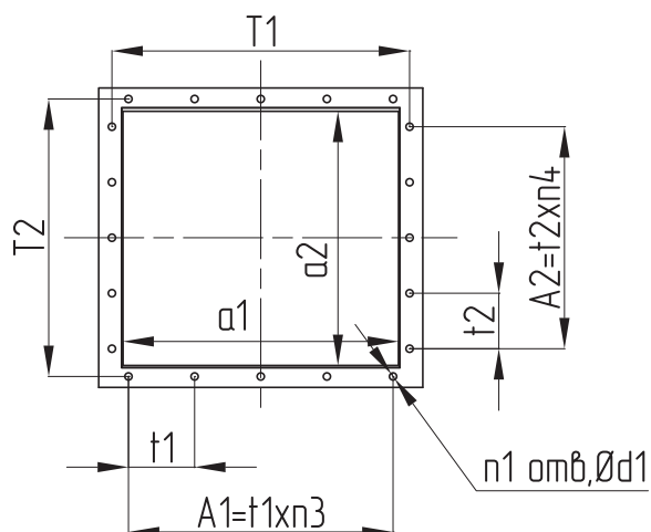
Выходной фланец
