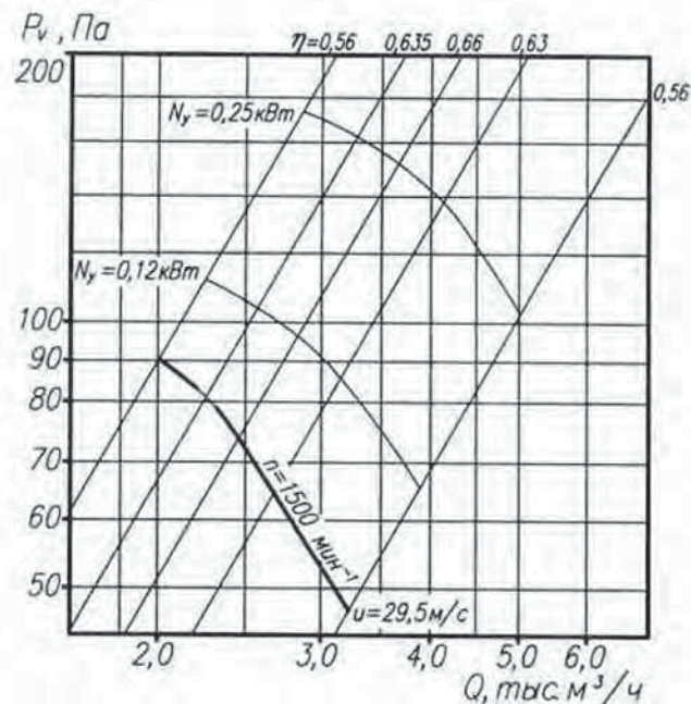
Аэродинамическая характеристика вентилятора ВО 06-300 №4
