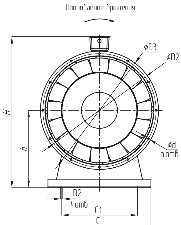
Компоновка 02
