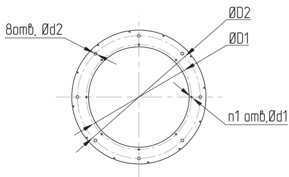
ВКР-ДУ 3.55...7.1
