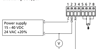
Схема проводки
