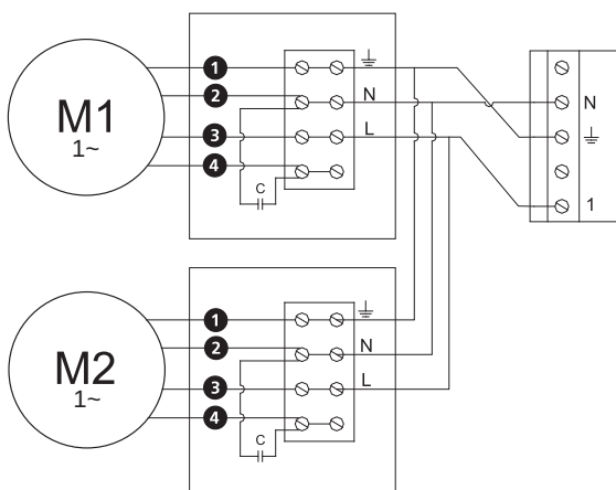
4040021 Однофазная с двумя радиальными вентиляторами с двусторонним всасыванием Однофазная с двумя двойными выходами отверстиями радиального вентилятора
