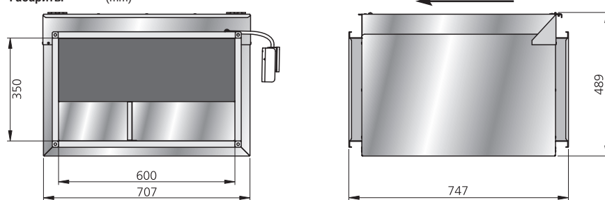
Технические данные
