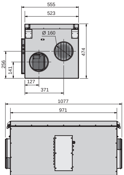
Габариты (mm)
