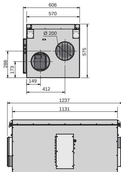
Габариты (mm)
