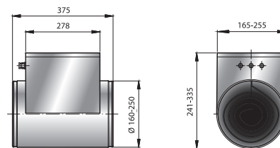
Размеры (мм)
