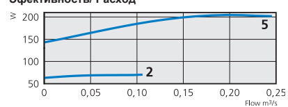
Эффективности/ Расход
