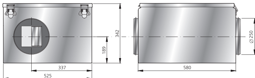
Габариты (mm)
