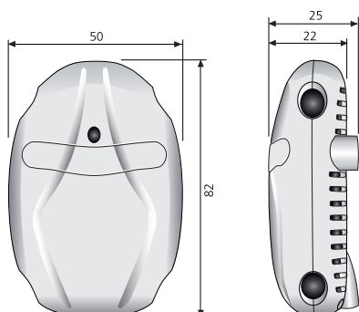
Размеры (мм)
