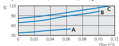
Потребляемая мощности/Расход воздуха
