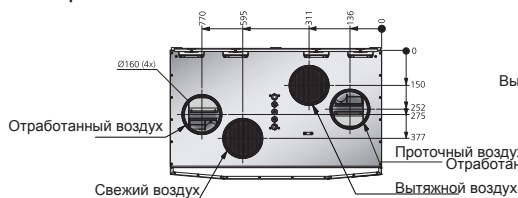
Левое исполнение
