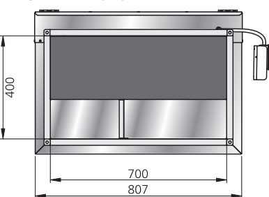
Технические данные
