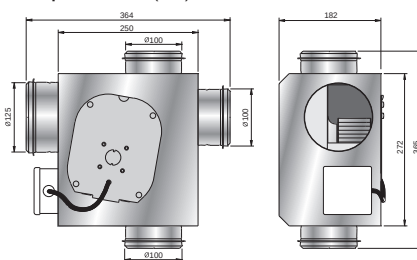
Габариты (mm)
