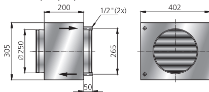
Размеры (мм)
