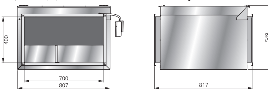
Технические данные
