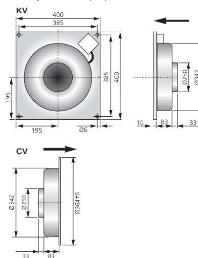
Габариты (mm)
