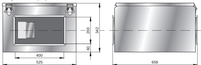
Габариты (mm)
