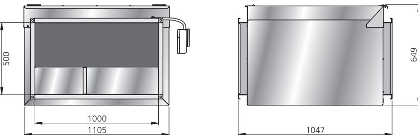
Технические данные
