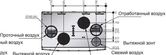
Левое исполнение с подключением вытяжного кухонного зонта
