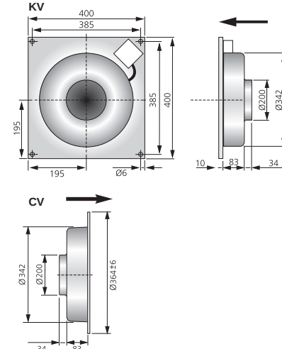
Габариты (mm)
