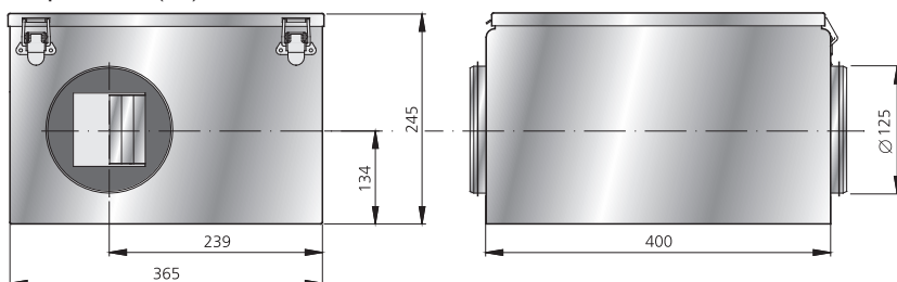
Габариты (mm)
