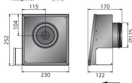
Габариты (mm)
