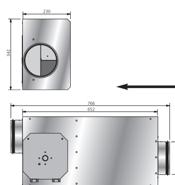
Габариты (mm)
