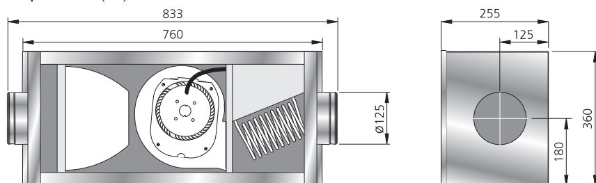
Габариты (mm)
