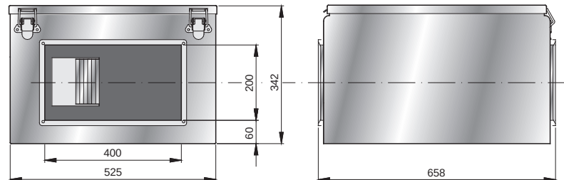
Габариты (mm)
