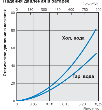
Падения давления в батареях
