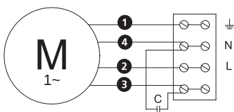
4040021 Однофазная с двумя радиальными вентиляторами с двусторонним всасыванием Однофазная с двумя двойными выходами отверстиями радиального вентилятора
