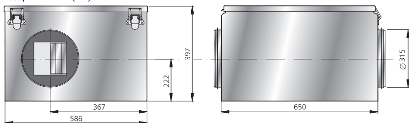
Габариты (mm)
