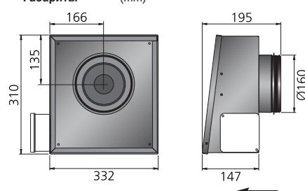
Габариты (mm)
