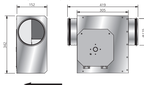
Габариты
