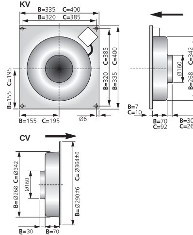
Габариты (mm)
