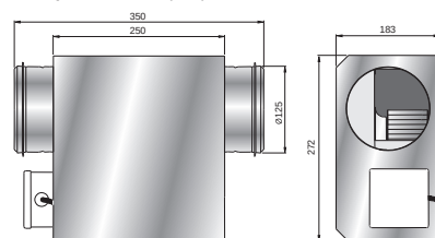
Габариты (mm)
