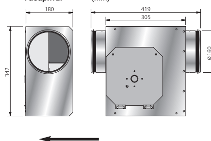
Габариты
