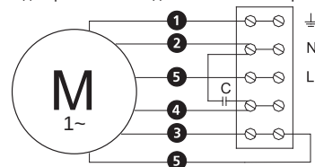
4040021 Однофазная с двумя радиальными вентиляторами с двусторонним всасыванием Однофазная с двумя двойными выходами отверстиями радиального вентилятора
