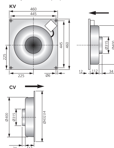
Габариты (mm)
