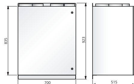
Габариты (mm)
